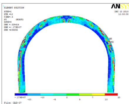
(a) Stresses ( Sy \times 10^{-2} MPa)
